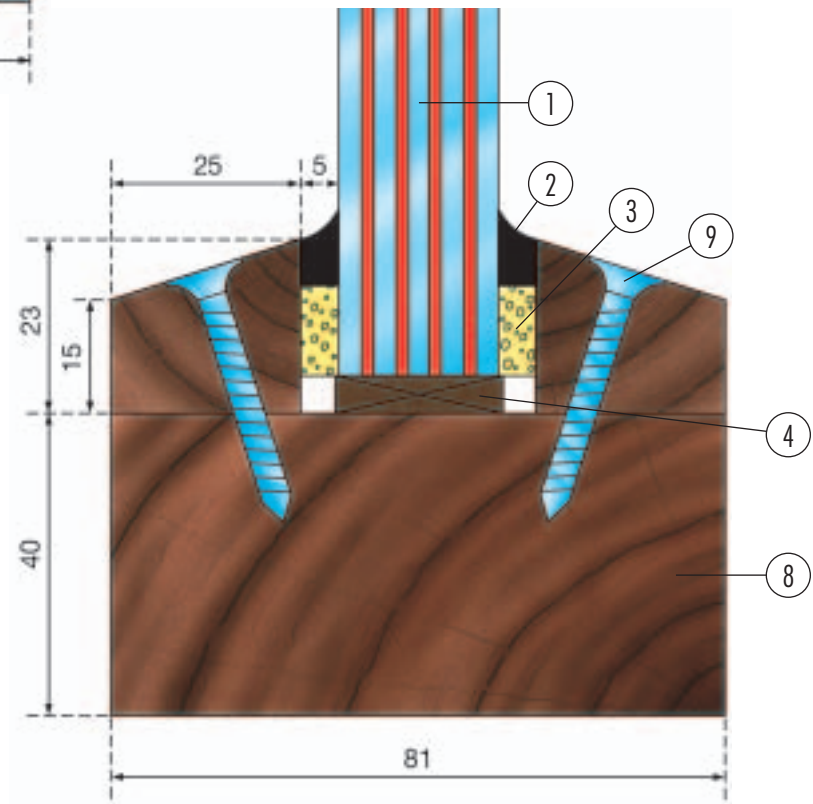
LPC TE 81342, LPC 340 suurused (mm)
